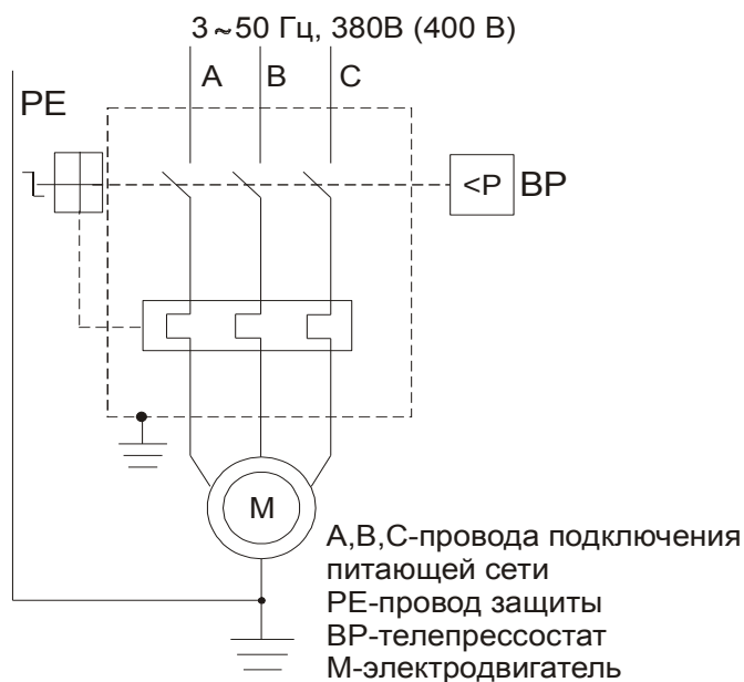
Рисунок 2 – Схема электрическая принципиальная
