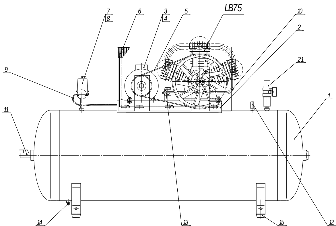
Рисунок 3 – Общий вид компрессора СБ4/Φ-270.LB75B
