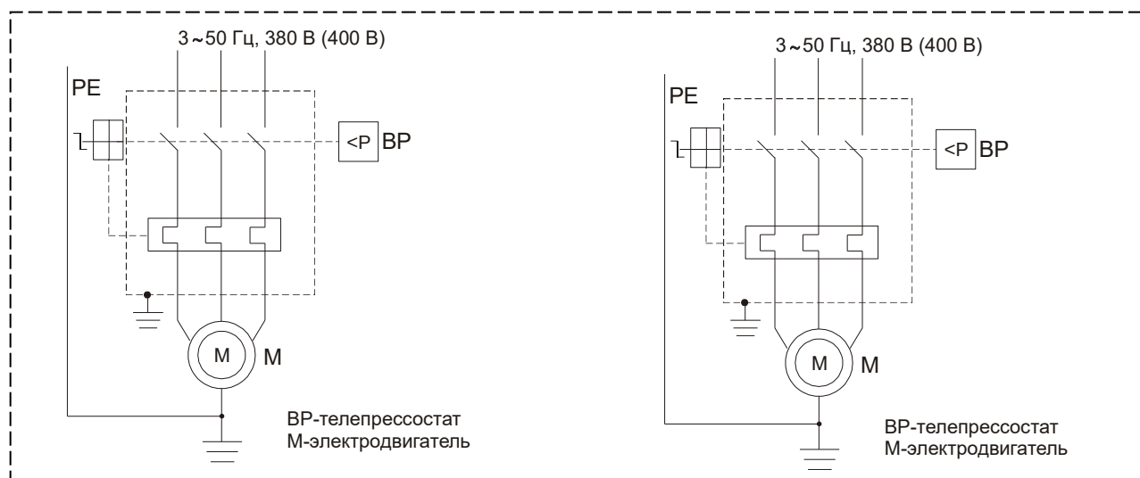
Рисунок 7 – Схема электрическая принципиальная для СБ4/Ф-500.LB75ТБ
