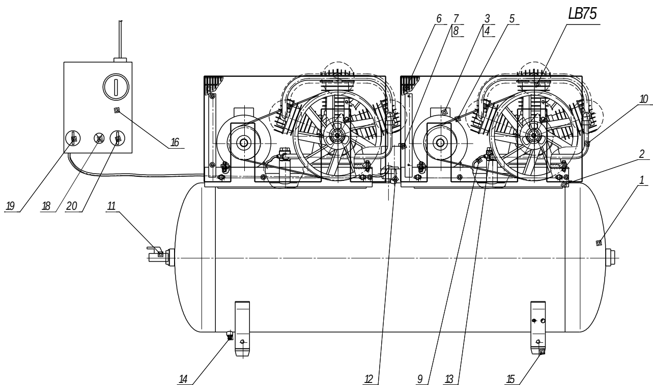
Рисунок 5 – Общий вид компрессора СБ4/Φ-500.LB75T
