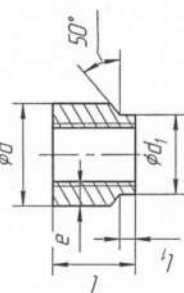
Деталь шпильки поз. 7
